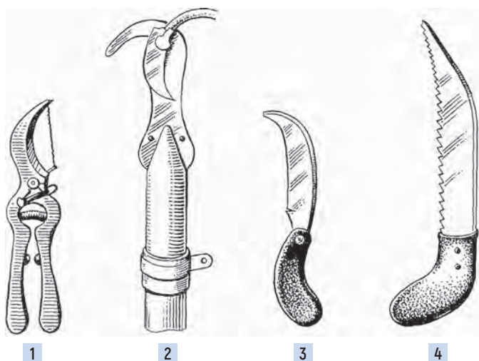
Инструменты для обрезки деревьев: 1 – секатор; 2 – сучкорез (воздушный секатор); 3 – садовый нож; 4 – ножовка садовая.
